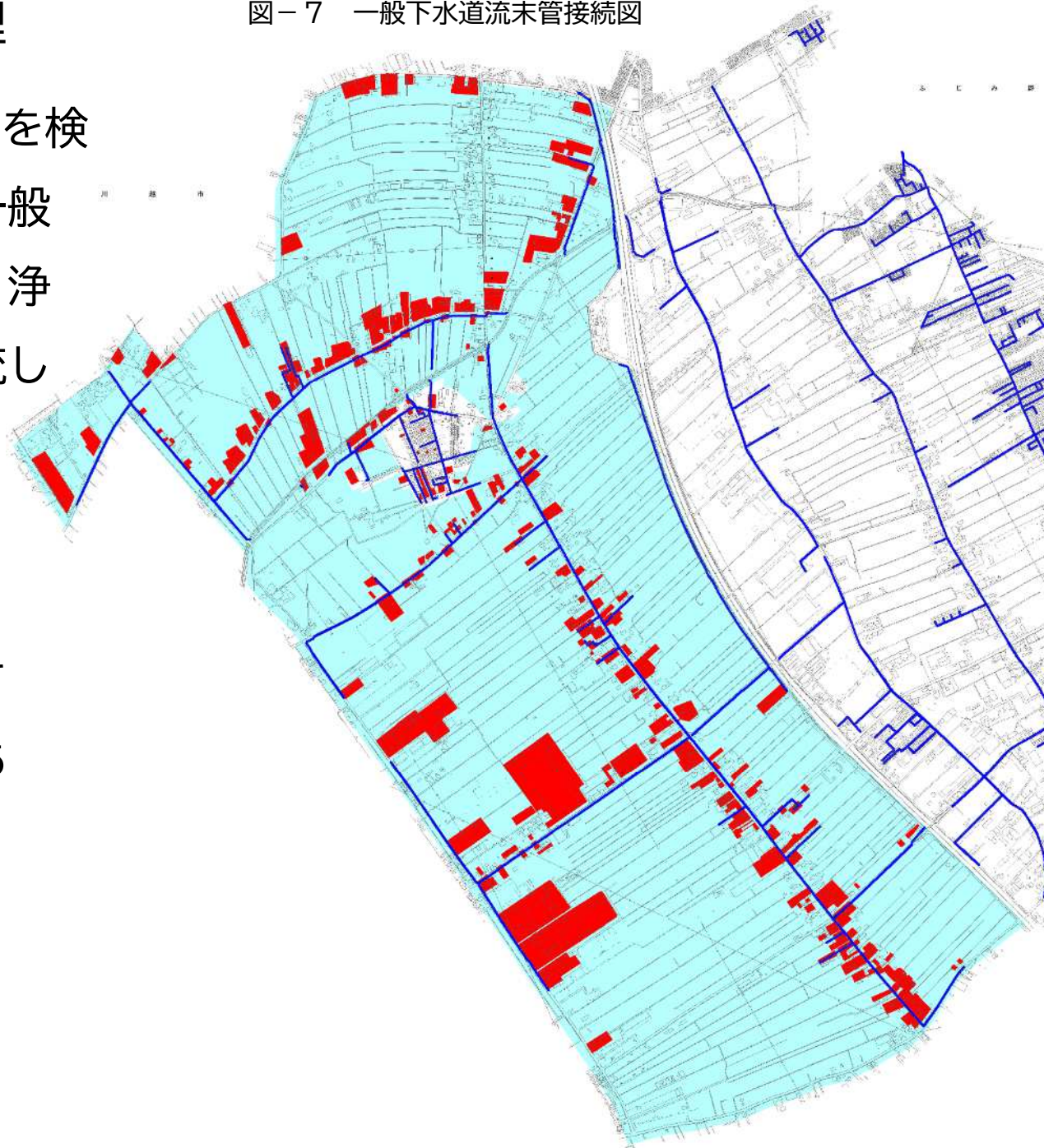
図-7 一般下水道流末管接続図
