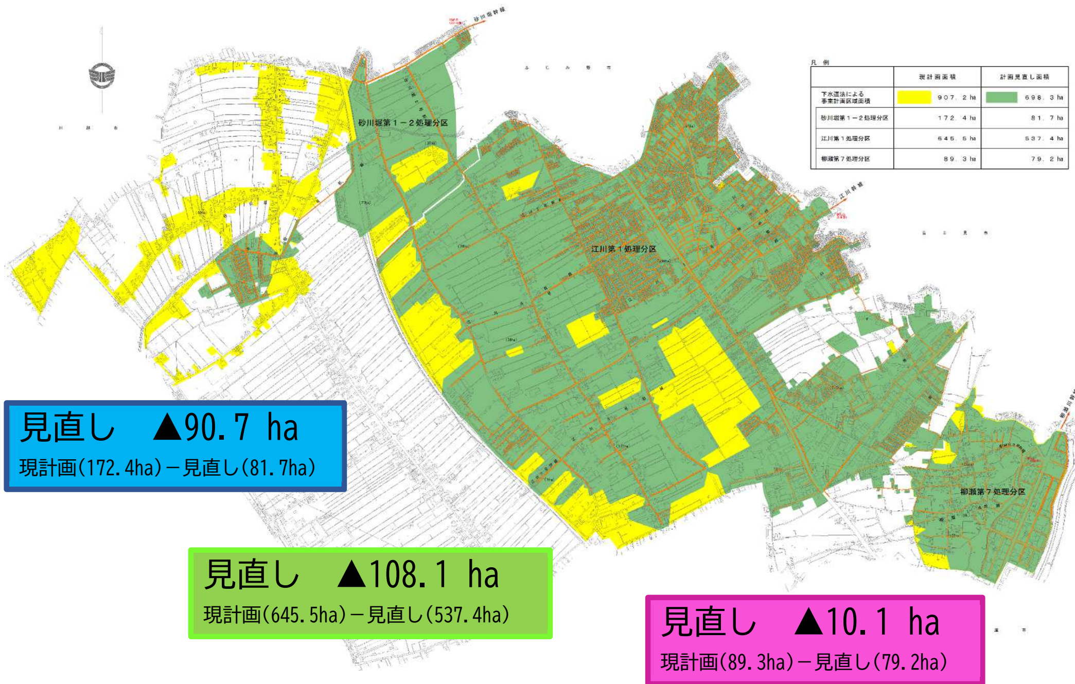
図-6 三芳町公共下水道事業計画見直し図
