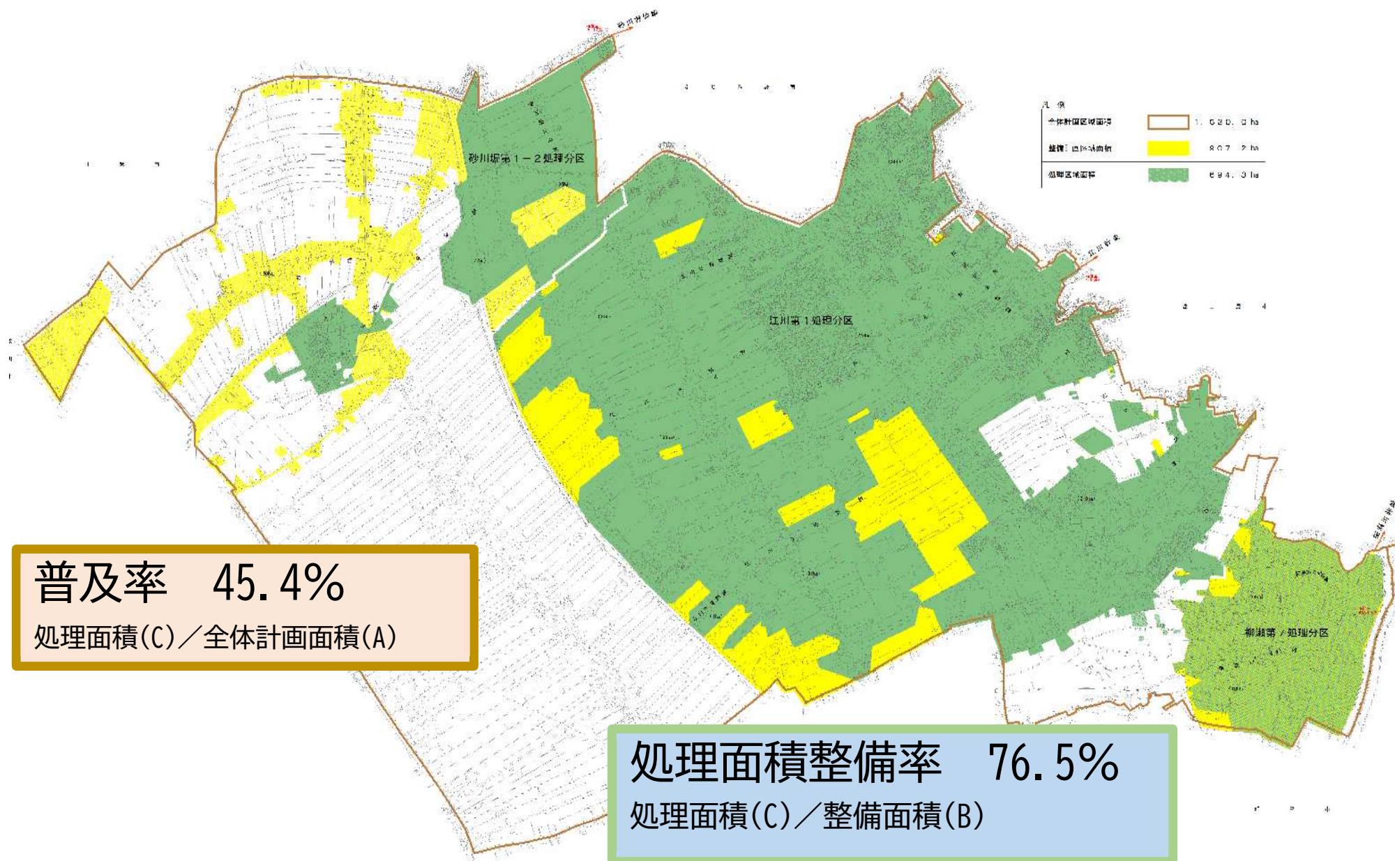
荒川右岸流域関連三芳公共下水道 整備状況
