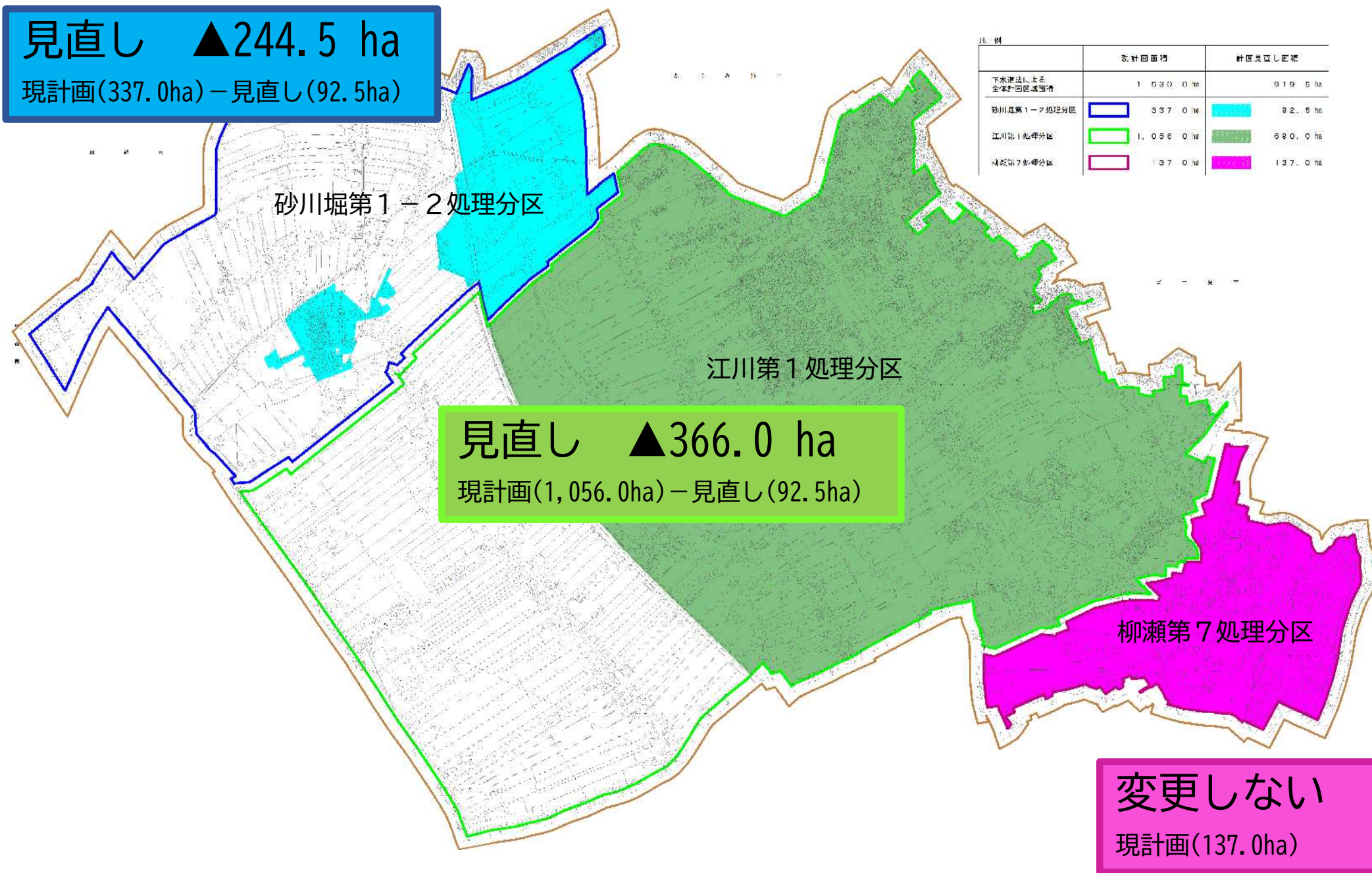
荒川右岸流域関連三芳公共下水道 全体計画見直し図
