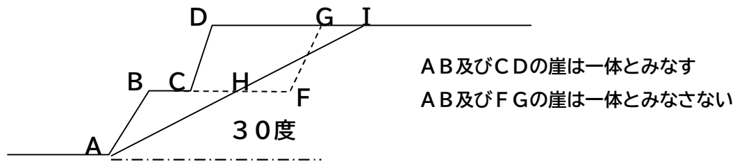
図－６ 一体の崖とみなす崖
