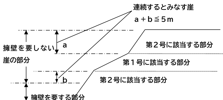
図－５ 擁壁を要しない崖又は崖の部分（４）
